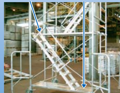
アルミ内階段手摺 踊場付
