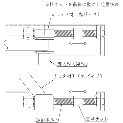
【立上げ装置】詳細
