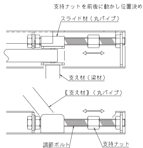
【立上げ装置】詳細
