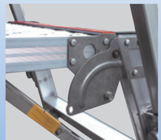
ステンレス材の導入拡大で軽量化。ガタつきを押さえる効果もあり。
